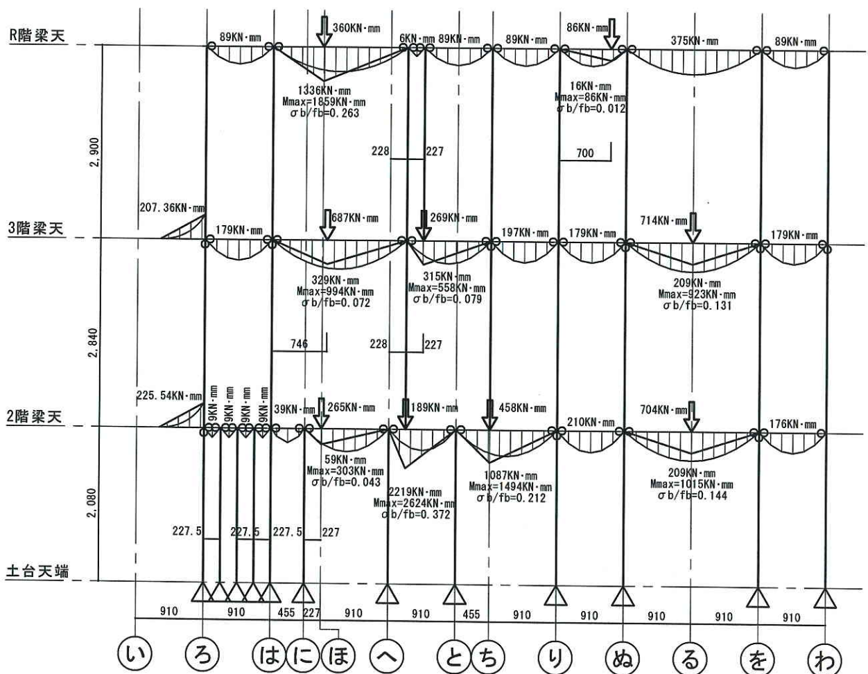
1通 短期応力図
