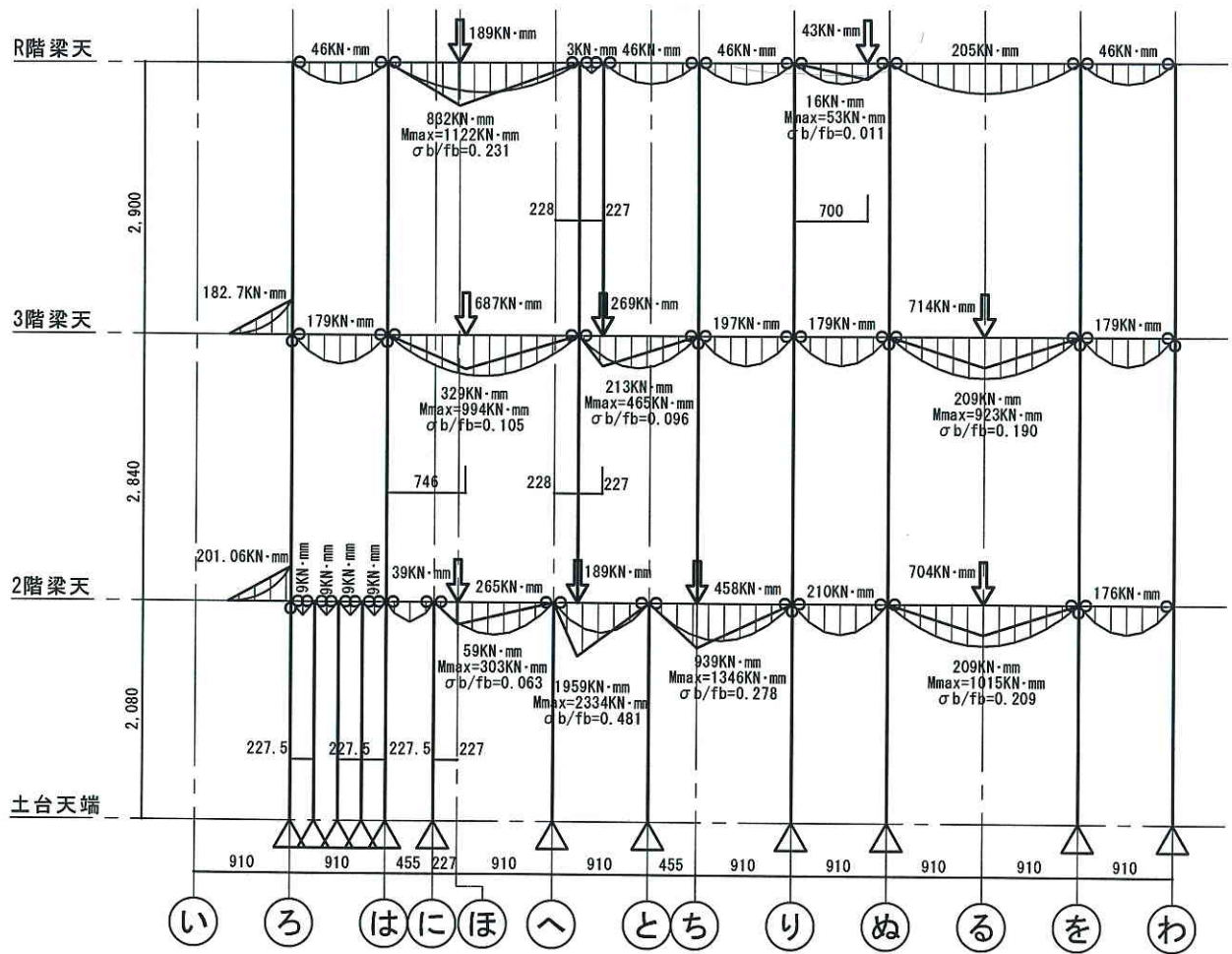
1通 長期応力図
