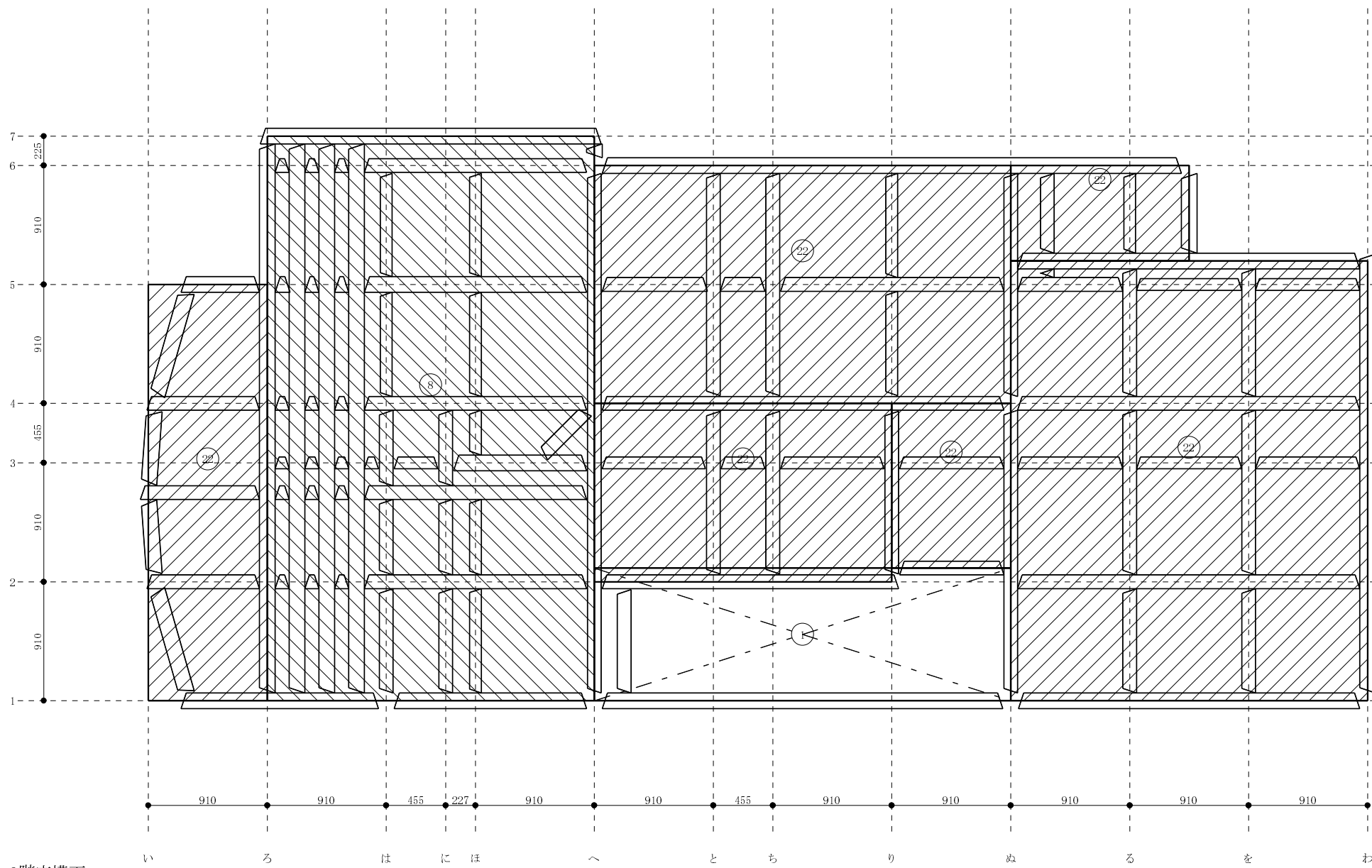
2階床構面
