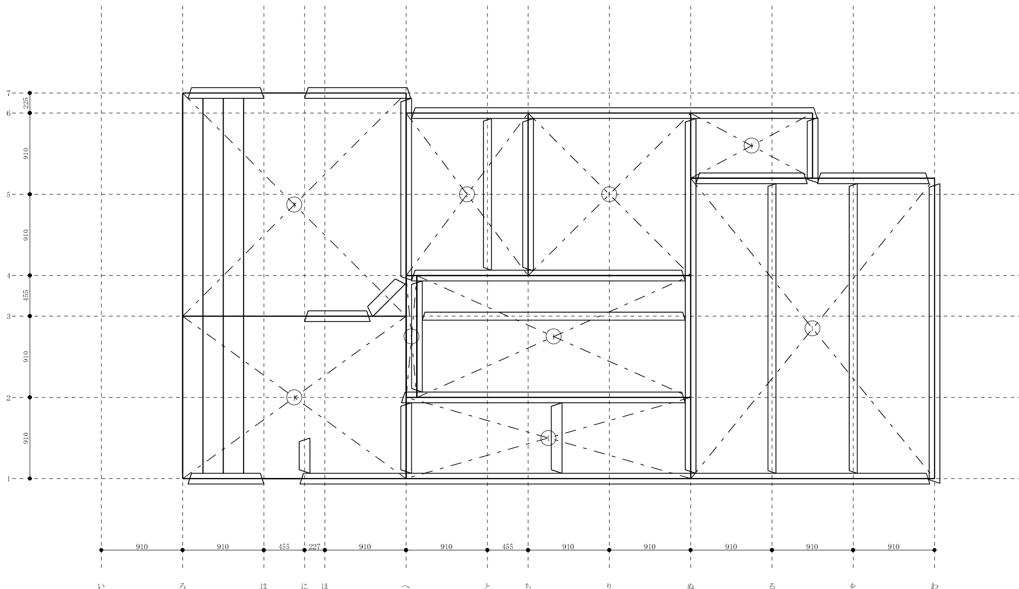
1階床構面
