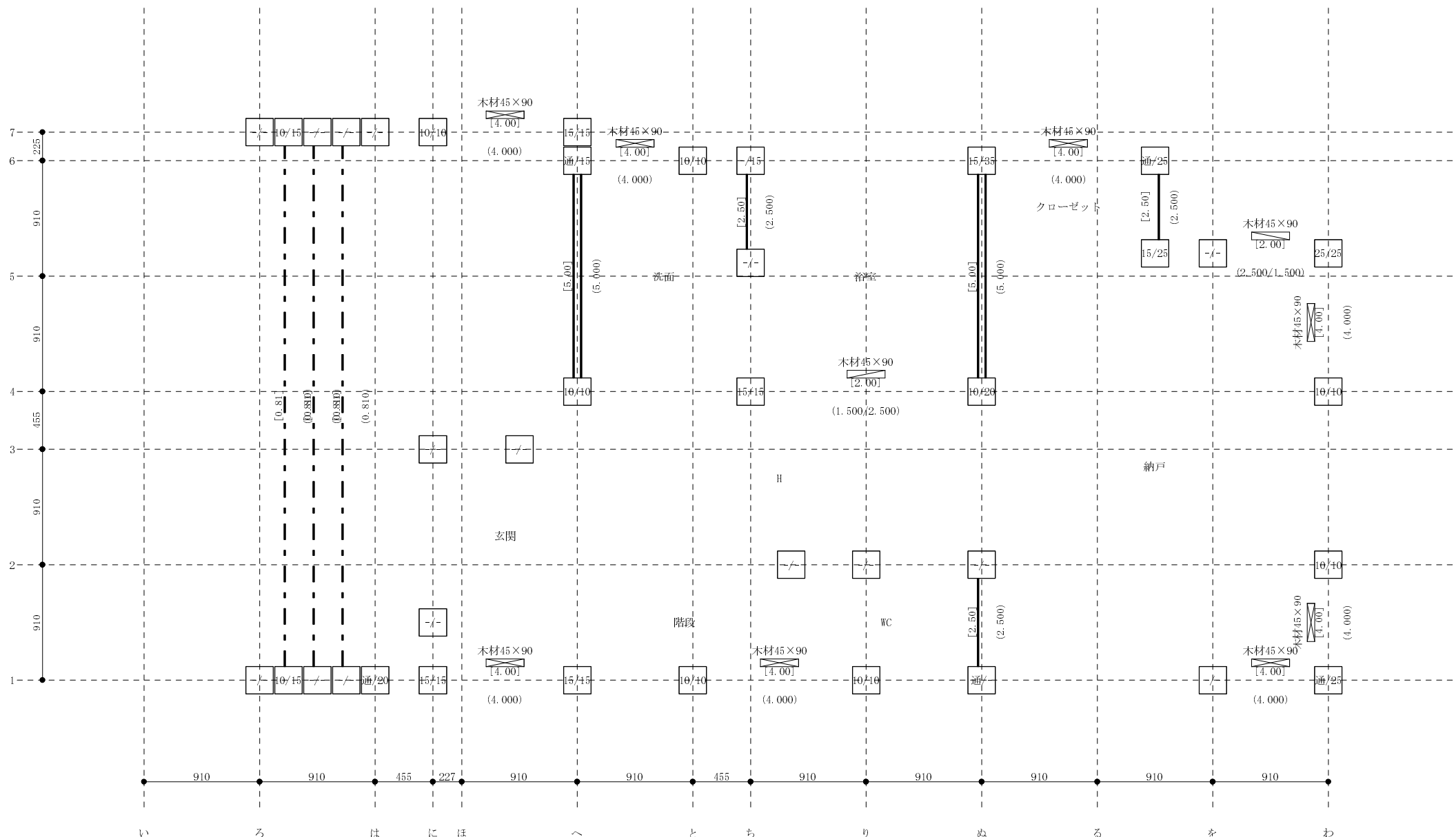
1階 柱壁伏図
