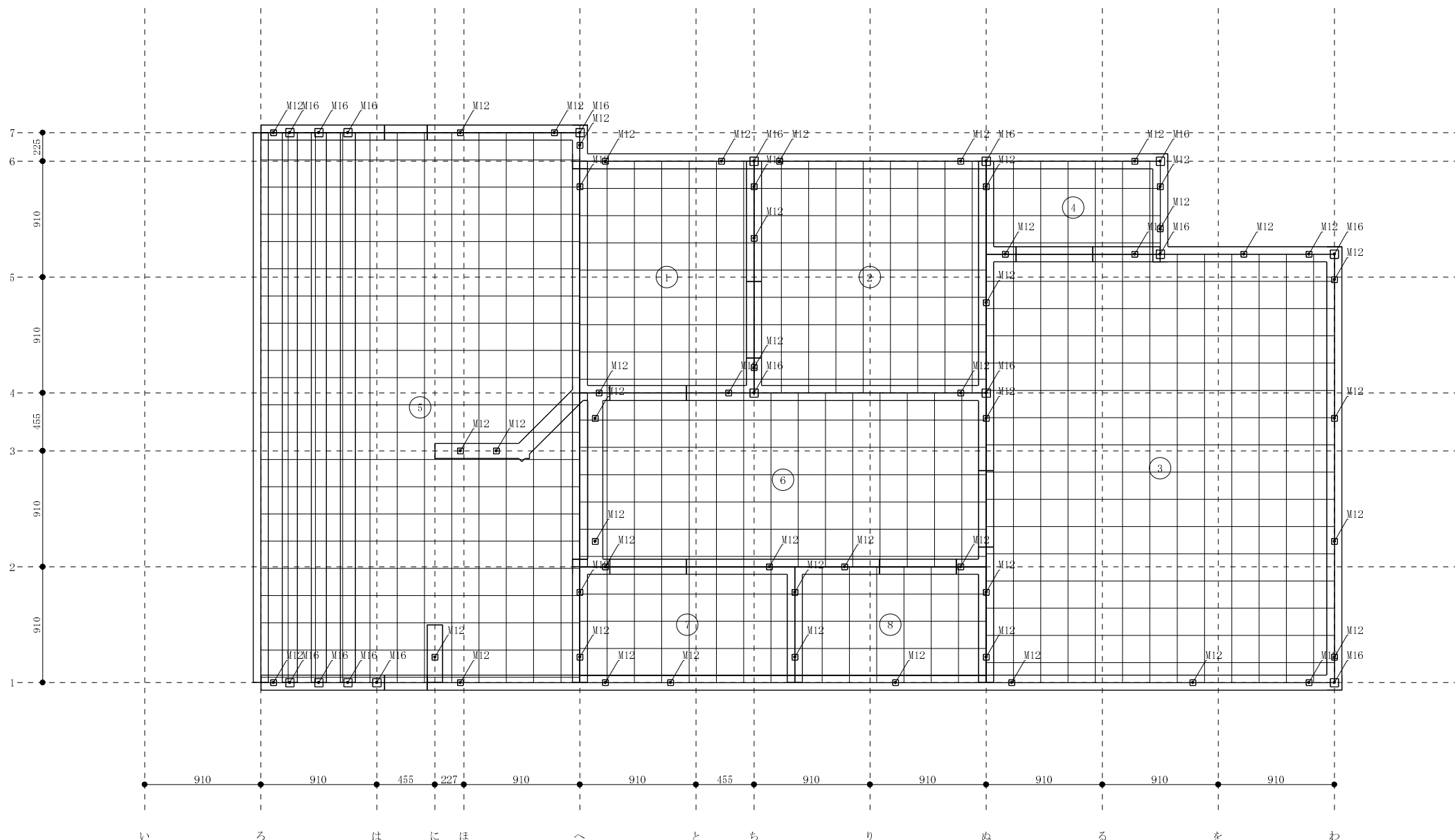
基礎伏図
