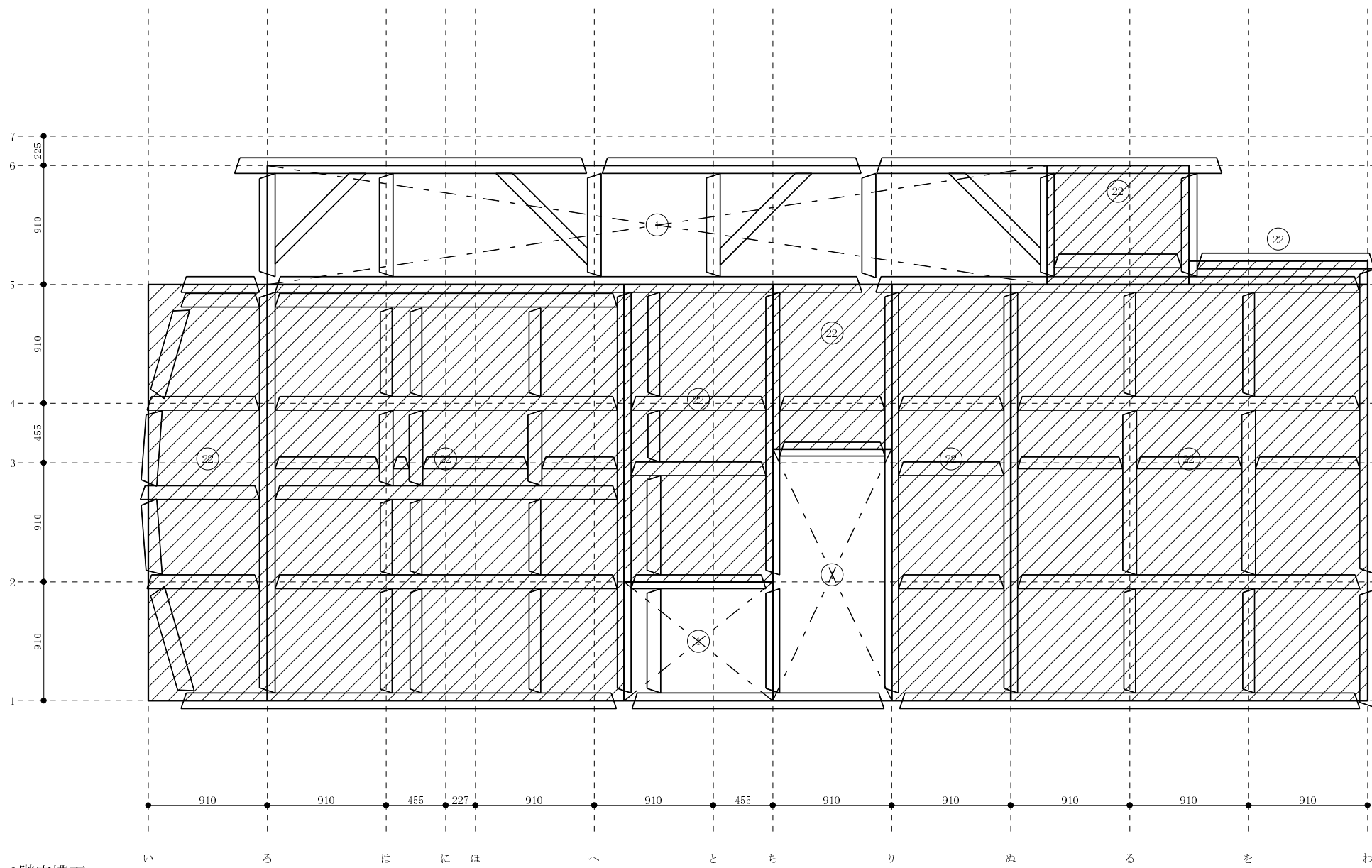
3階床構面
