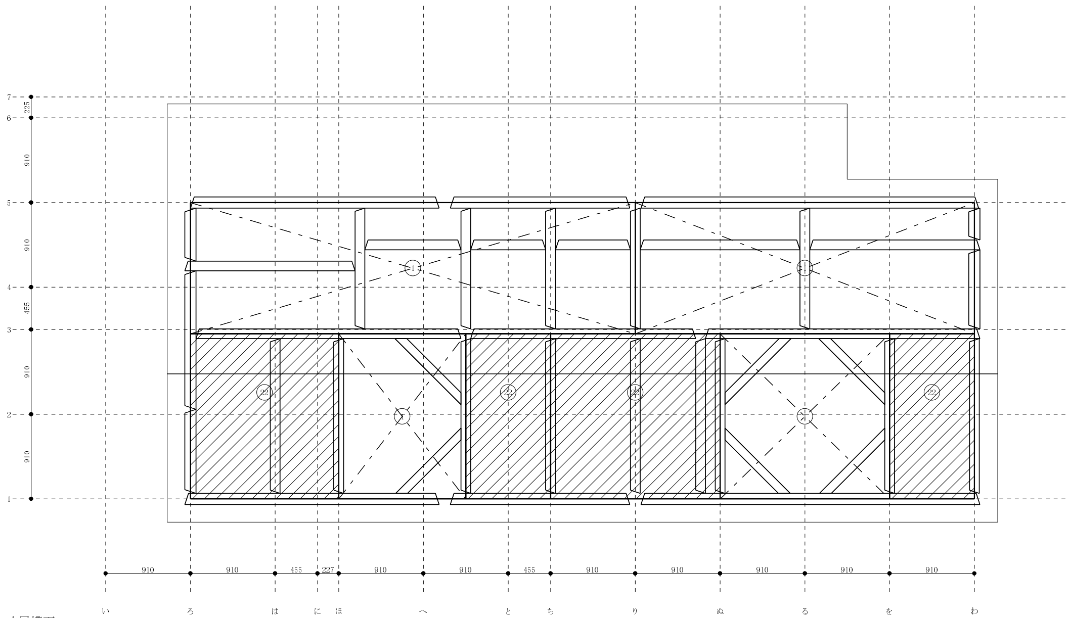
小屋構面
