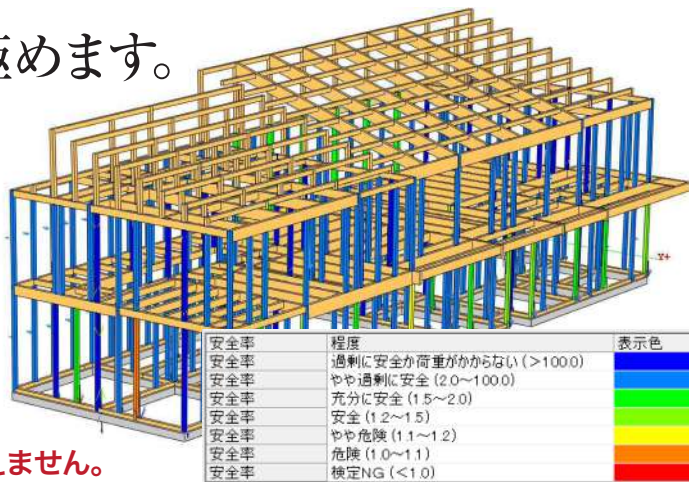
部材の安全率(危険度)は、色分けして表示。
